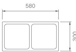
12. skrivbordslåda djup 2 cm desk drawer depth 2 cm
