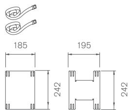
10. datorhållare pc holder
