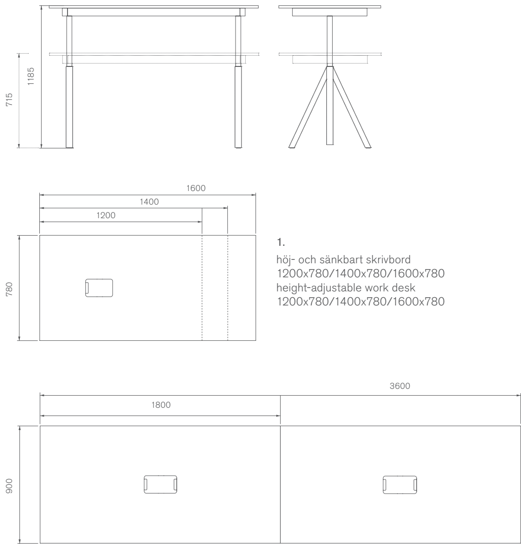
1. høj- og sænkbart skrivebord 1200x780/1400x780/1600x780 height-adjustable work desk 1200x780/1400x780/1600x780 2. høj- og sænkbart møtesbord 1800x900 høj- og sænkbart konferensbord 3600x900 height-adjustable meeting table 1800x900 height-adjustable conference table 3600x900
