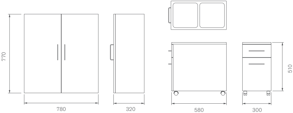
4. förvaringsskåp filing cabinet
