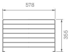
6. trådraster för skrivbord wire screen for desk
